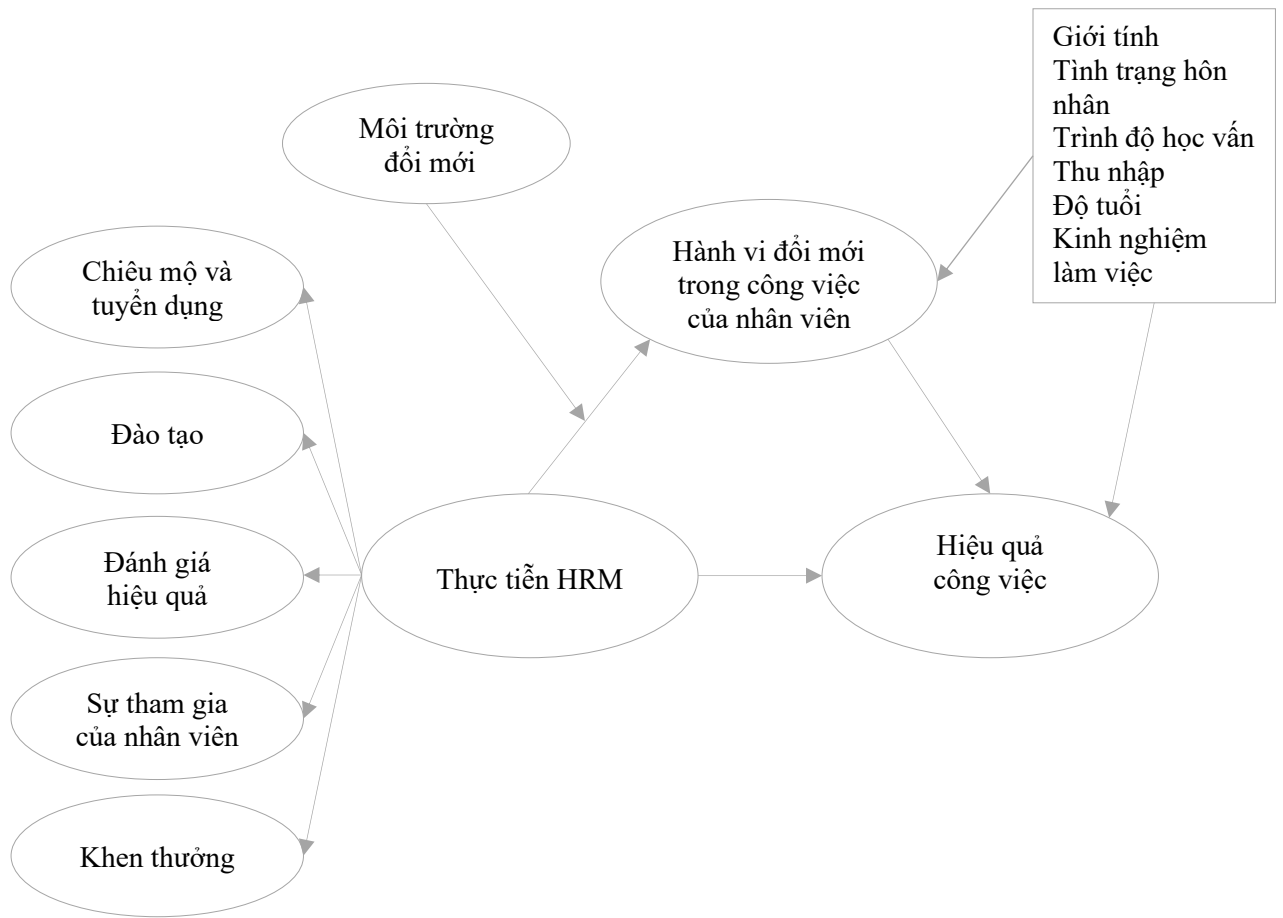
Hình 3.2. Mô hình nghiên cứu sau khi điều chỉnh
