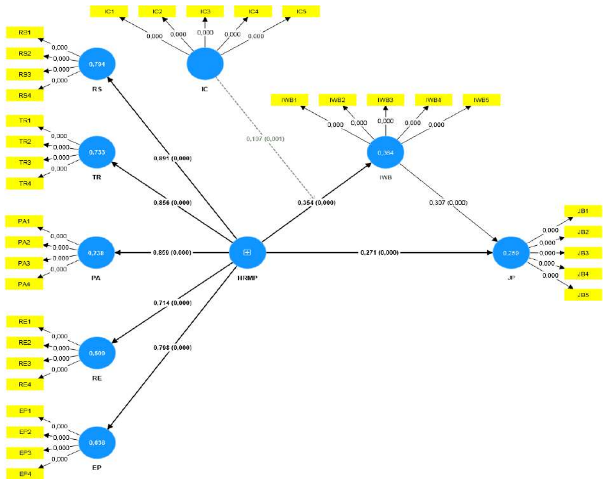
Hình 4.12. Mô hình cấu trúc PLS-SEM
